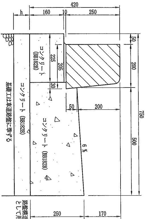
横断面図
