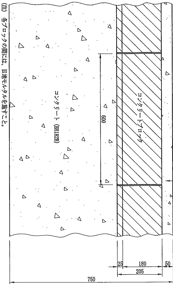
平面図
