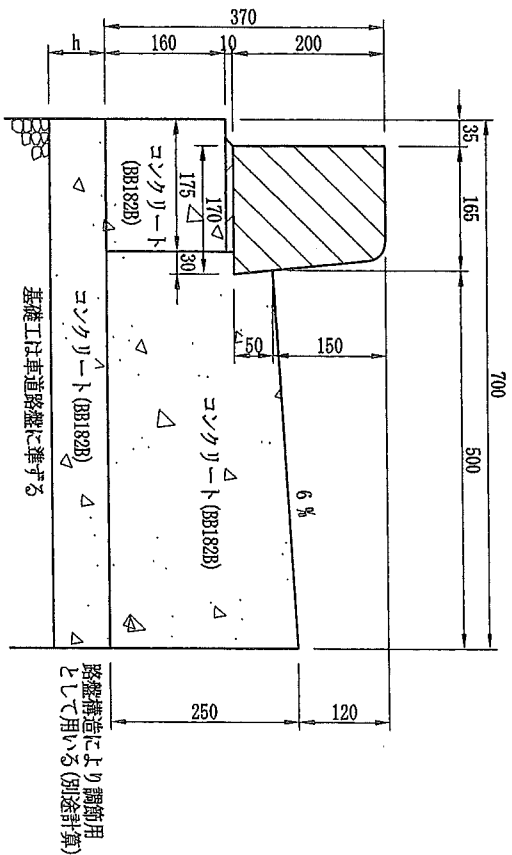
縦断面図
